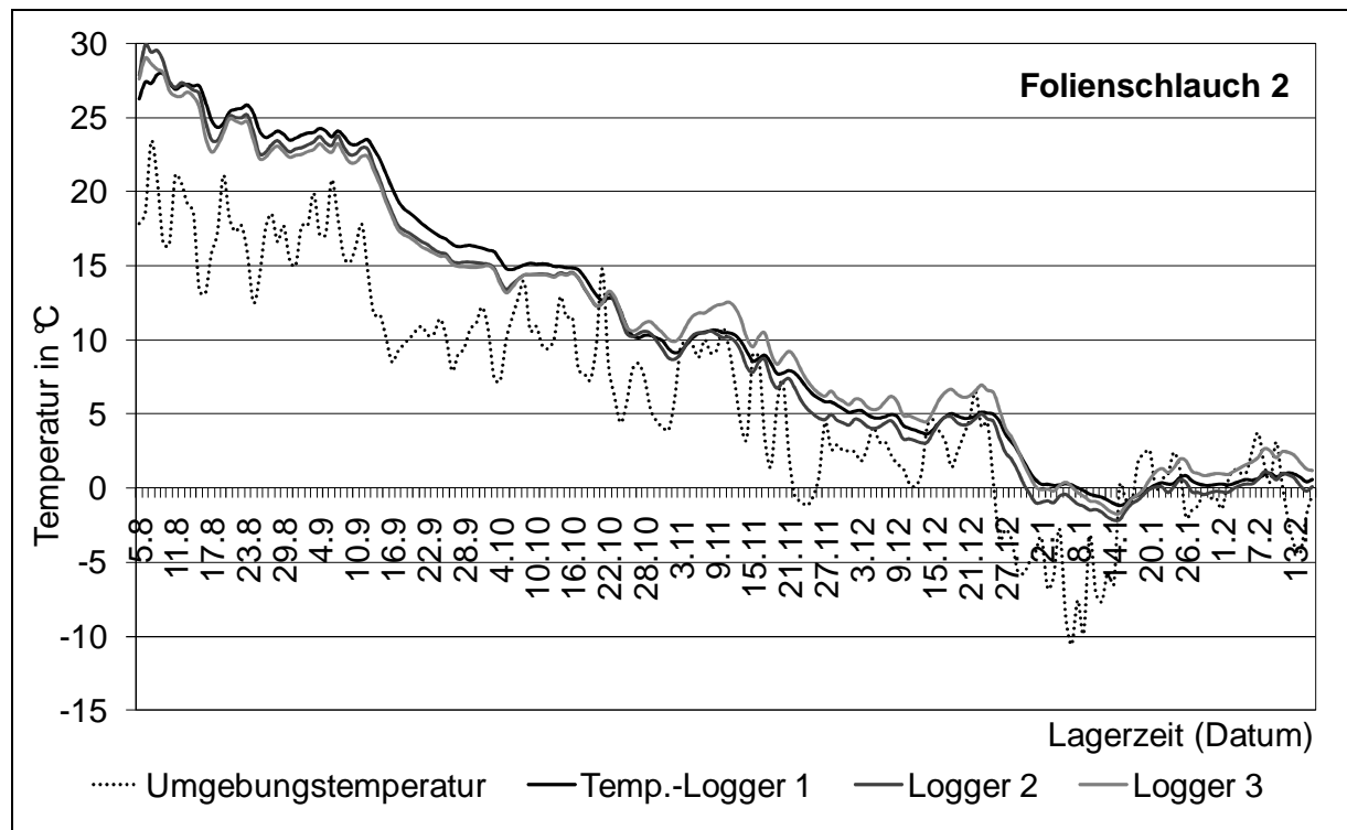
Abb. 10: Temperaturverlauf im Schlauch 2 und Außentemperatur über die Lagerdauer (WAGNER, IDLER, 2009)
