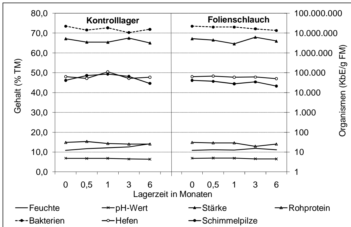
Abb. 11: Chemische und mikrobiologische Kennwerte von Weizen während der 6monatigen Lagerung in Kontrolllager und Folienschlauch (WAGNER, IDLER, 2009)
